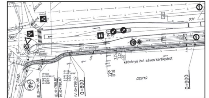
Litér-Balatonfűzfő kerékpárút B/2. engedélyezés alatt lévő szakasz-részlet
